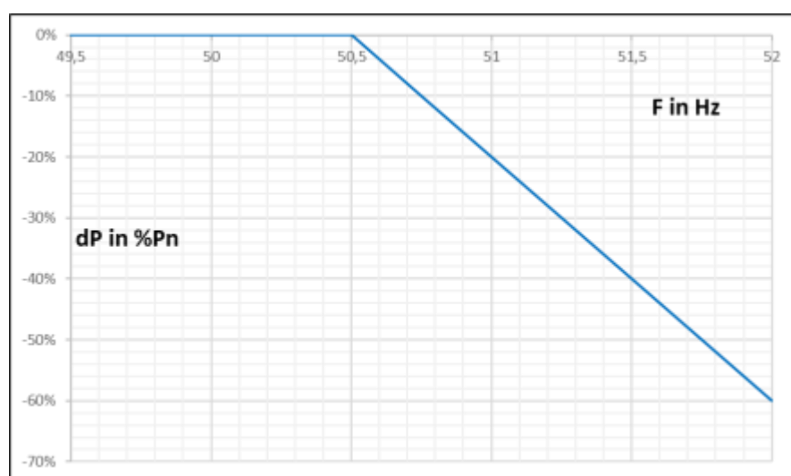
Figure 5 .- Réglage de Fréquence en cas de surfréquences
