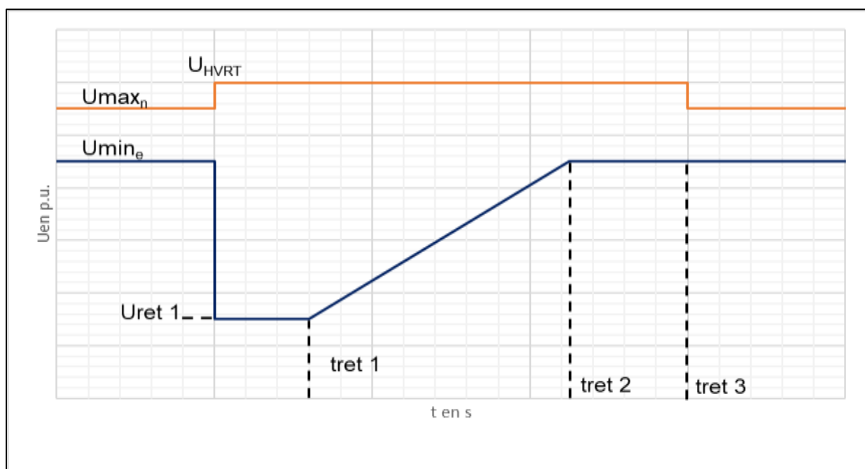
Figure 9 .- Profil de tenue aux Creux de Tension/surtension d'une Installation de Production à raccorder sur un réseau Basse Tension
