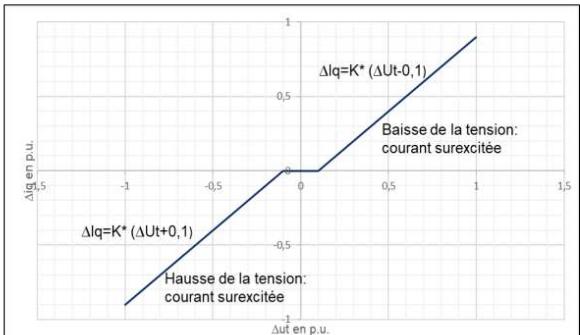
Figure 7.- Injection de courant réactif en fonction de la variation de tension en cas de Creux de Tension ou hausse de tension- Installations non synchrones
